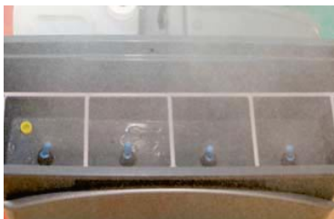
Vier justierbare Sprühdüsen.
