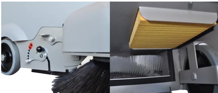
Sweep 41: Die Bürsthöhe ist schnell und leicht veränderbar.
