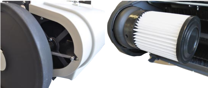
Als einzige mechanische Kehrmaschine verfügt die Sweep 5 plus über eine patentierter Absaugung mit einem Filter für Feinstaub.
