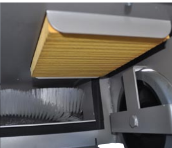
Der Staubfilter der Sweep 41 ist leicht zu wechseln und zu reinigen.
