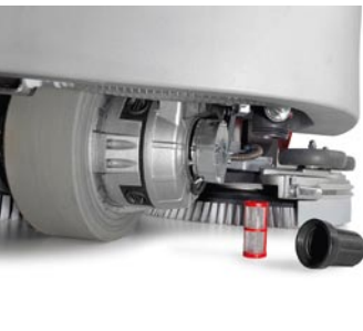
Hocheffiziente und starke Antriebsmotoren und gut zugängliche Frischwasserfilter.
