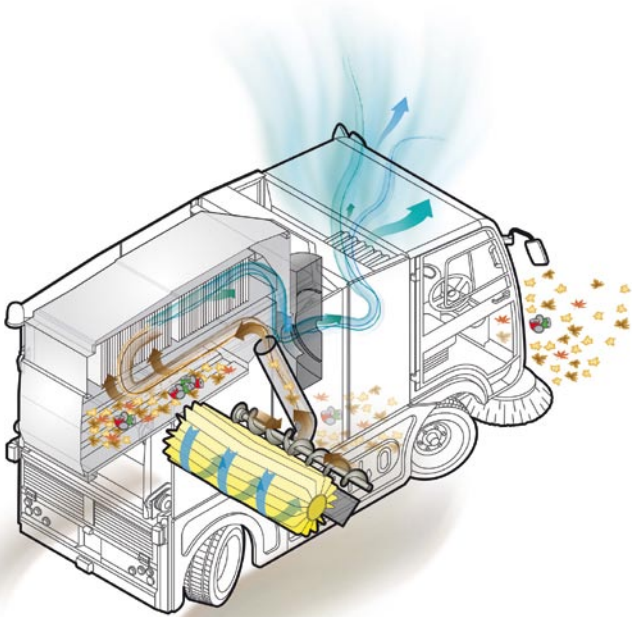
CS 140 Funktionsprinzip
