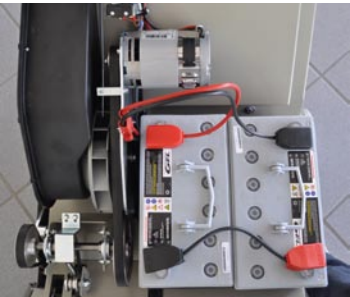
Sweep CS60 AB: Aufgeräumte, robuste Technik – Power durch moderne wartungsfreie Batterien.
