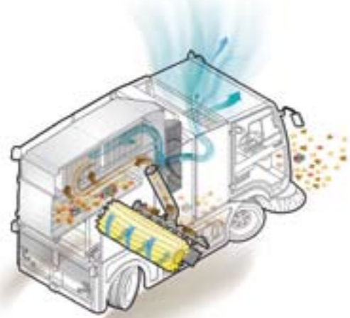
CS 140 Funktionsprinzip
